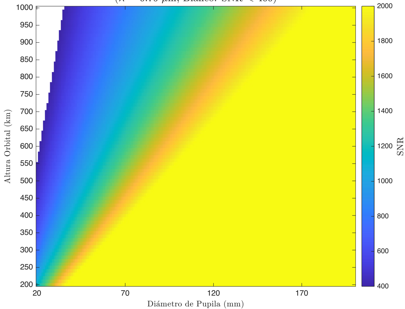
SNR - Cassegrain - Detector 3 ( \lambda = 0.76 \mu\text{m} , Blanco: SNR < 400)
